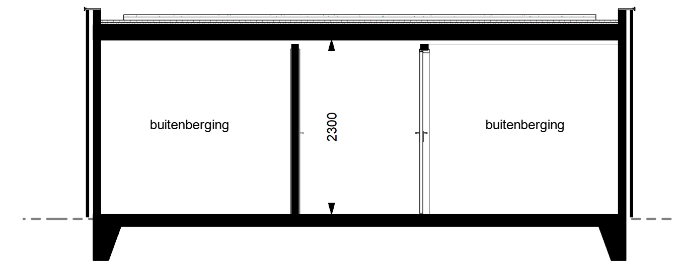
doorsnede Schaal: 1 : 50
